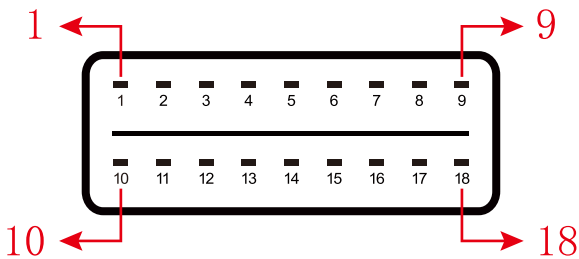
KDS3.1尿素泵侧接头针脚图
